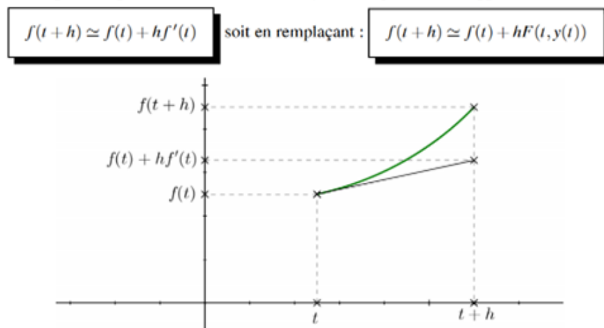
Figure 2. Méthode d'Euler explicite
