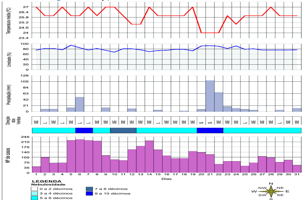
Figura 10 - Aracaju, Análise Rítmica do mês de maio do ano de 2008.
