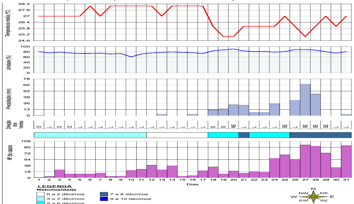
Figura 8 - Aracaju, Análise Rítmica do mês de março do ano de 2008.
