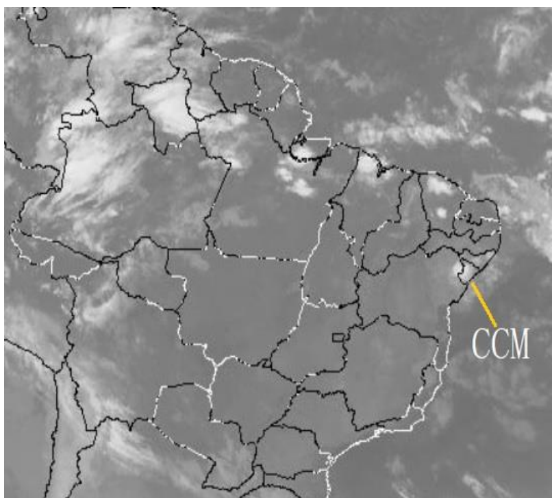
Figura 7 - Banda de nebulosidade por formação de CCM - 27/04/2001.
