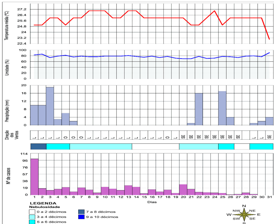
Figura 6 - Aracaju, Análises Rítmicas do mês de maio do ano de 2001.
