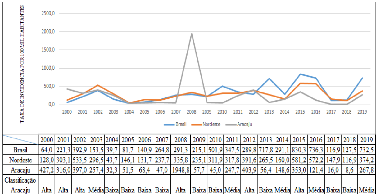
Figura 3 - Taxa de incidência de casos de dengue por 100 mil habitantes no Brasil, na região Nordeste e em Aracaju, no período de 2000 a 2019.
