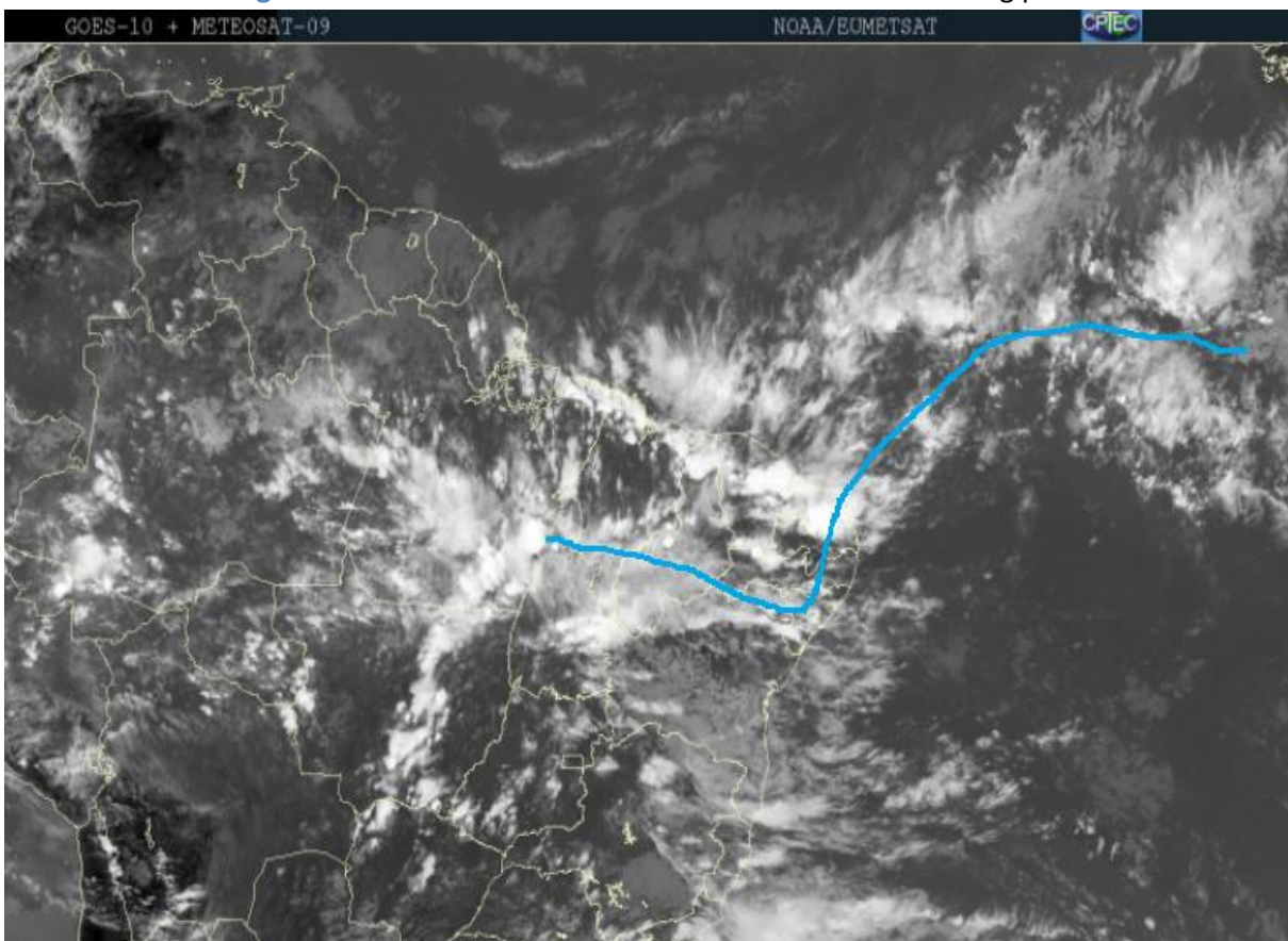
Figura 11 - Faixa de nebulosidade associada a ZCIT sobre Sergipe.
