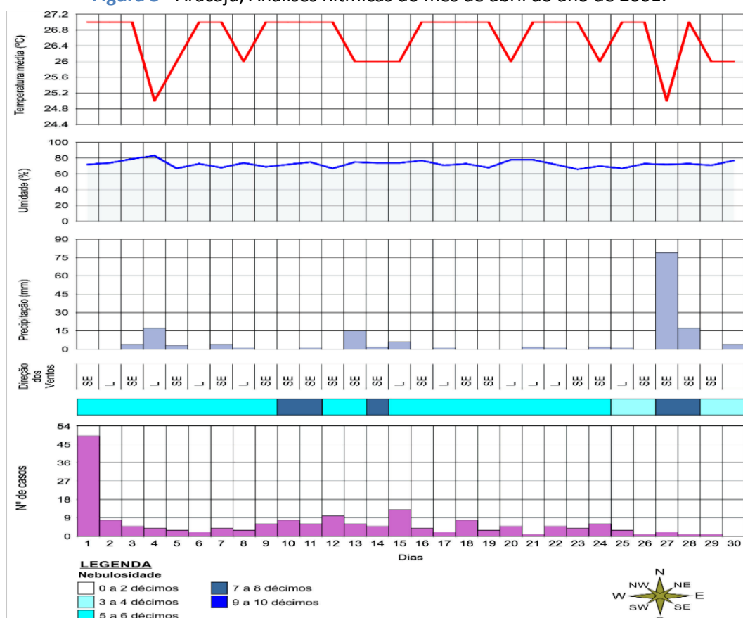
Figura 5 - Aracaju, Análises Rítmicas do mês de abril do ano de 2001.
