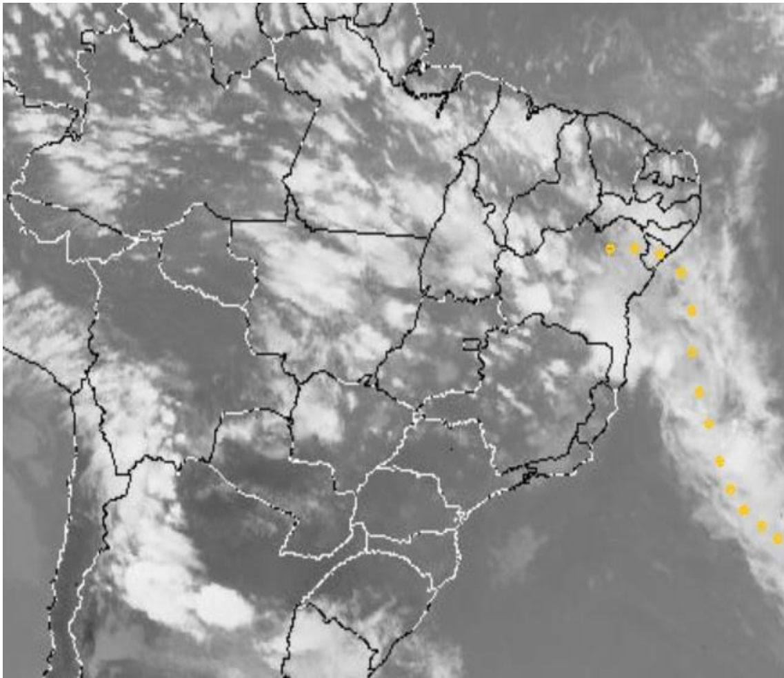
Figura 4 - Atuação da ZCAS sobre Aracaju/SE - 21/01/2000.
