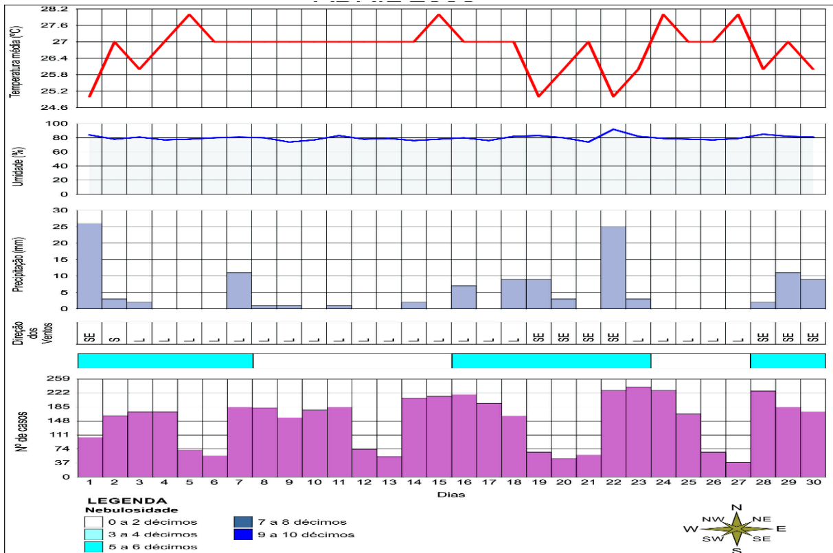
Figura 9 - Aracaju, Análise Rítmica do mês de abril do ano de 2008.
