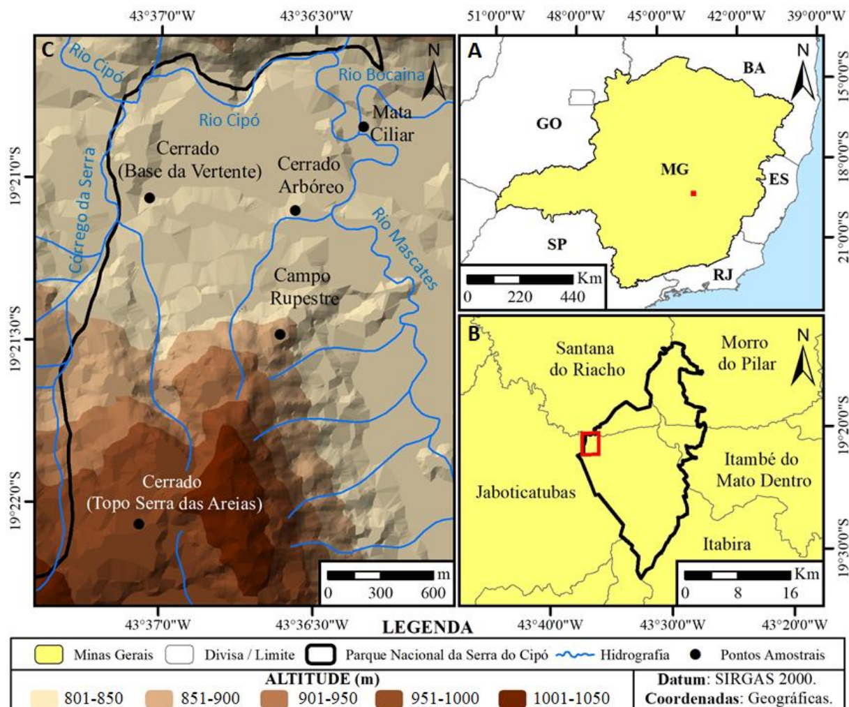
Figura 1 - Localização do Parque Nacional da Serra do Cipó no estado de Minas Gerais (A), limites do parque e municípios adjacentes com destaque em vermelho para a área de estudo aproximada (B), ampliada à esquerda com elementos da altimetria e hidrografia (C). Fontes:
