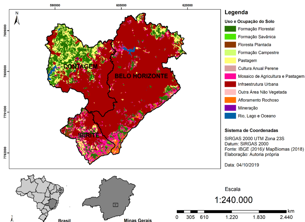
Figura 8 - Uso e Ocupação do Solo na área de estudo. Fonte: Autora deste, 2019.
