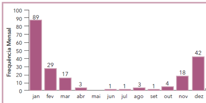
Figura 6 - Frequência mensal de deslizamentos de massa no Estado de Minas Gerais, no período de 1991 a 2012. Fonte: Atlas Brasileiro de Desastres Naturais, 2013.
