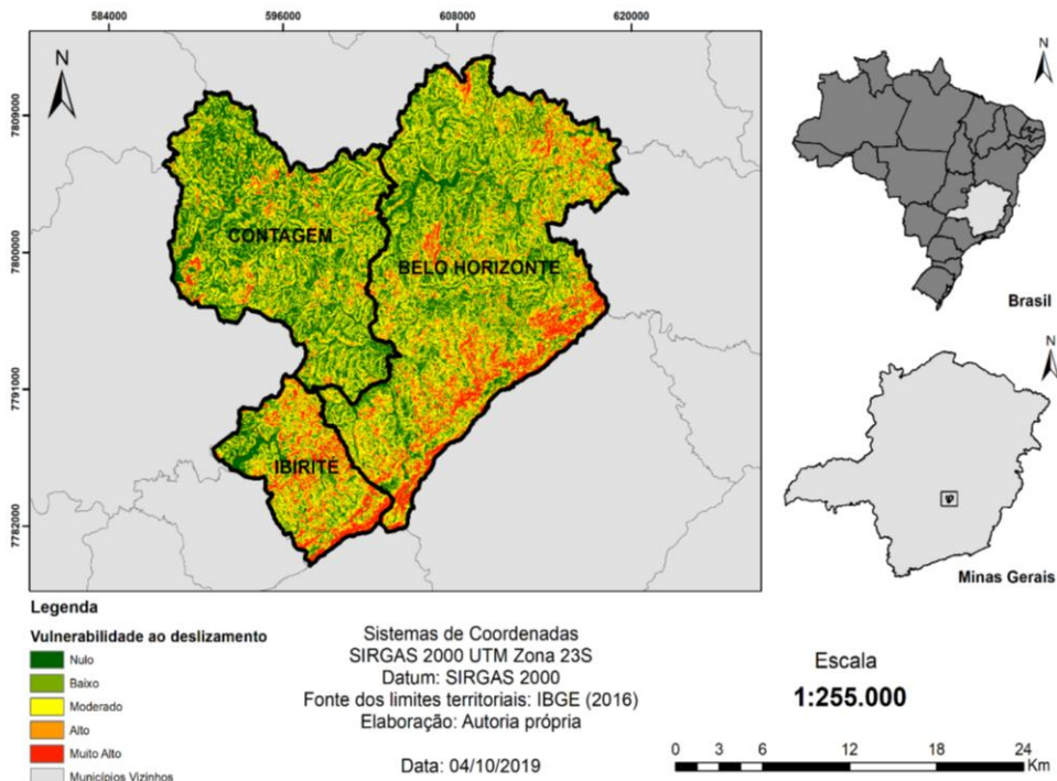
Figura 9 - Mapa de vulnerabilidade ao deslizamento de massa. Fonte: Autora deste, 2019.
