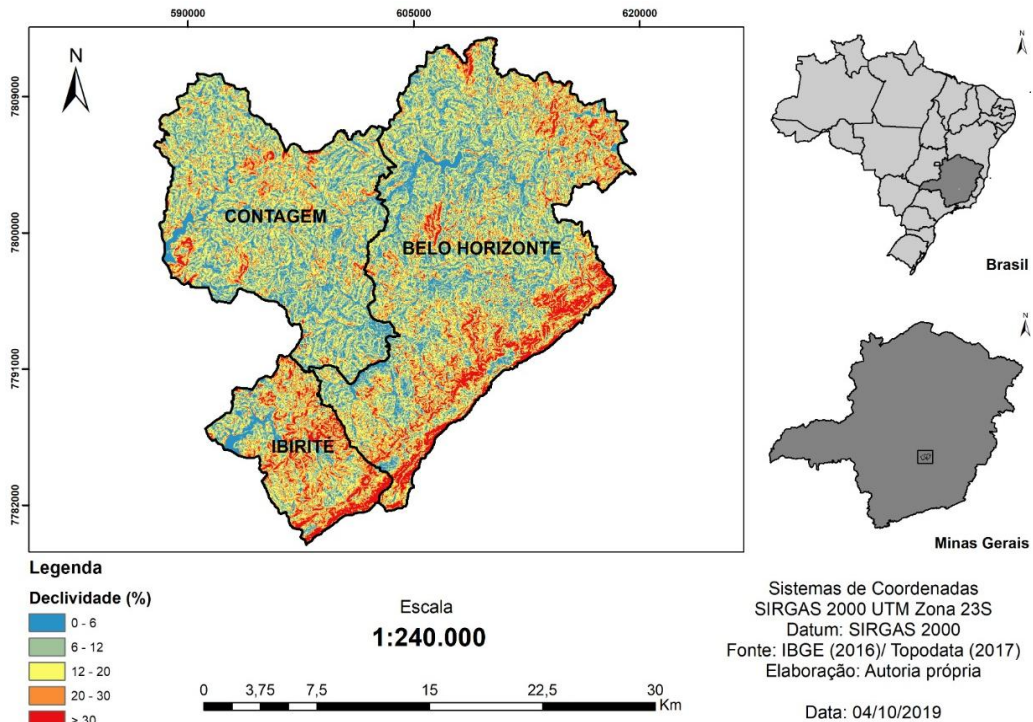
Figura 7 - Declividade do terreno na área de estudo. Fonte: Autora deste, 2019.
