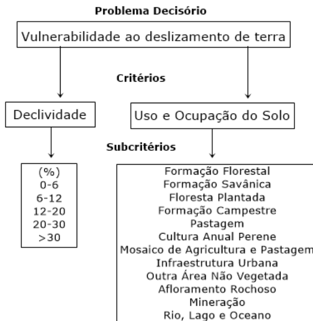
Figura 2 - Ordem Hierárquica do problema. Fonte: Autora deste, 2019.
