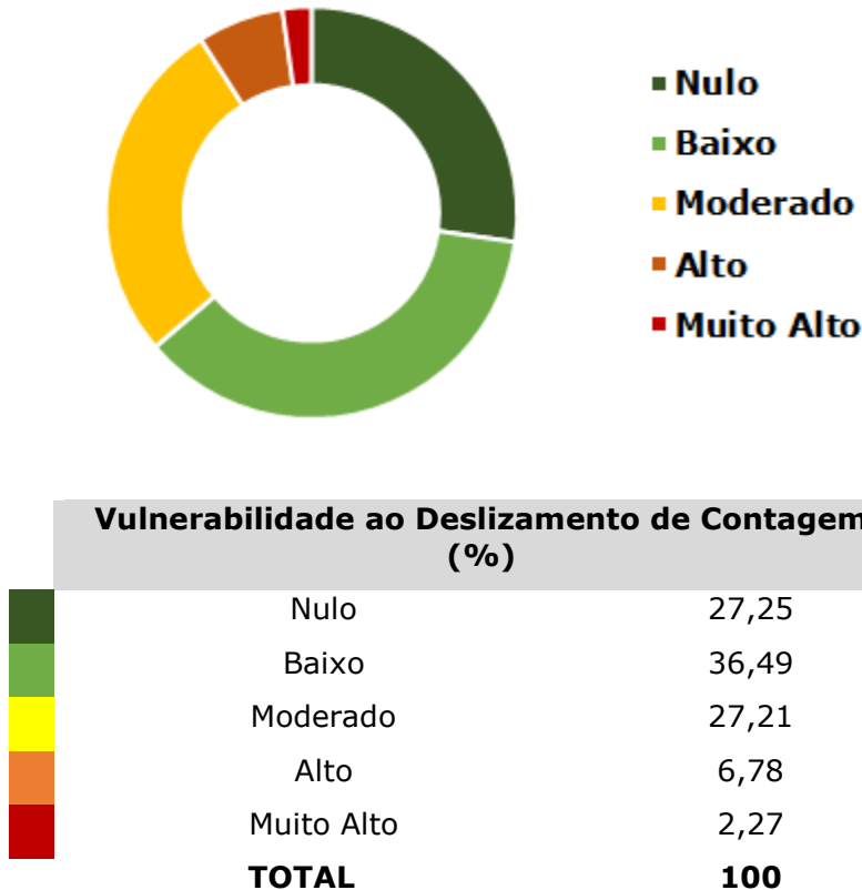
Figura 12 - Porcentagem de vulnerabilidade ao deslizamento em Contagem Fonte: Autora deste, 2019.
