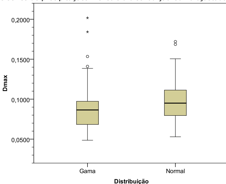
Figura 2 - Box-Plots dos valores de D_{max} do teste de Kolmogorov-Smirnov para a aderência das séries de precipitações anuais a distribuição Gama e Normal.
