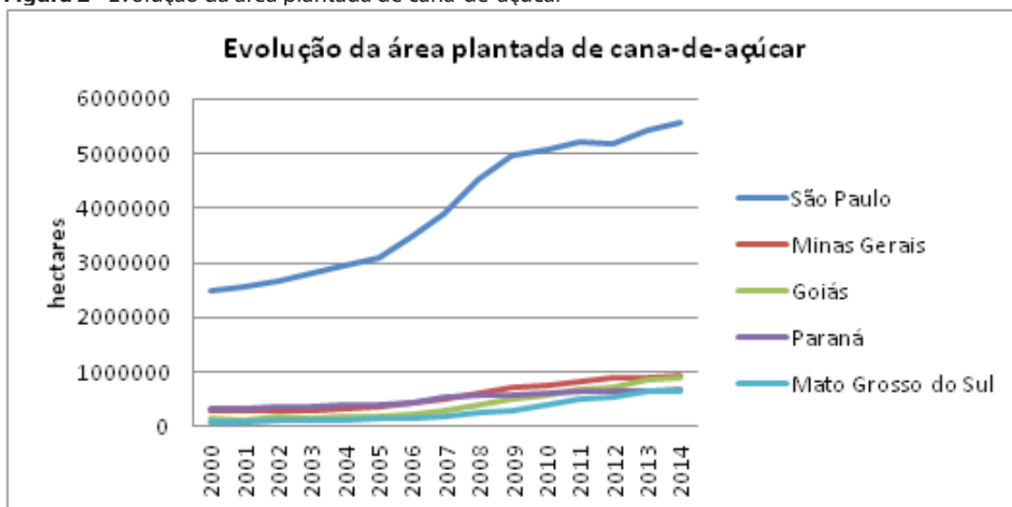
Figura 2 - Evolução da área plantada de cana-de-açúcar
