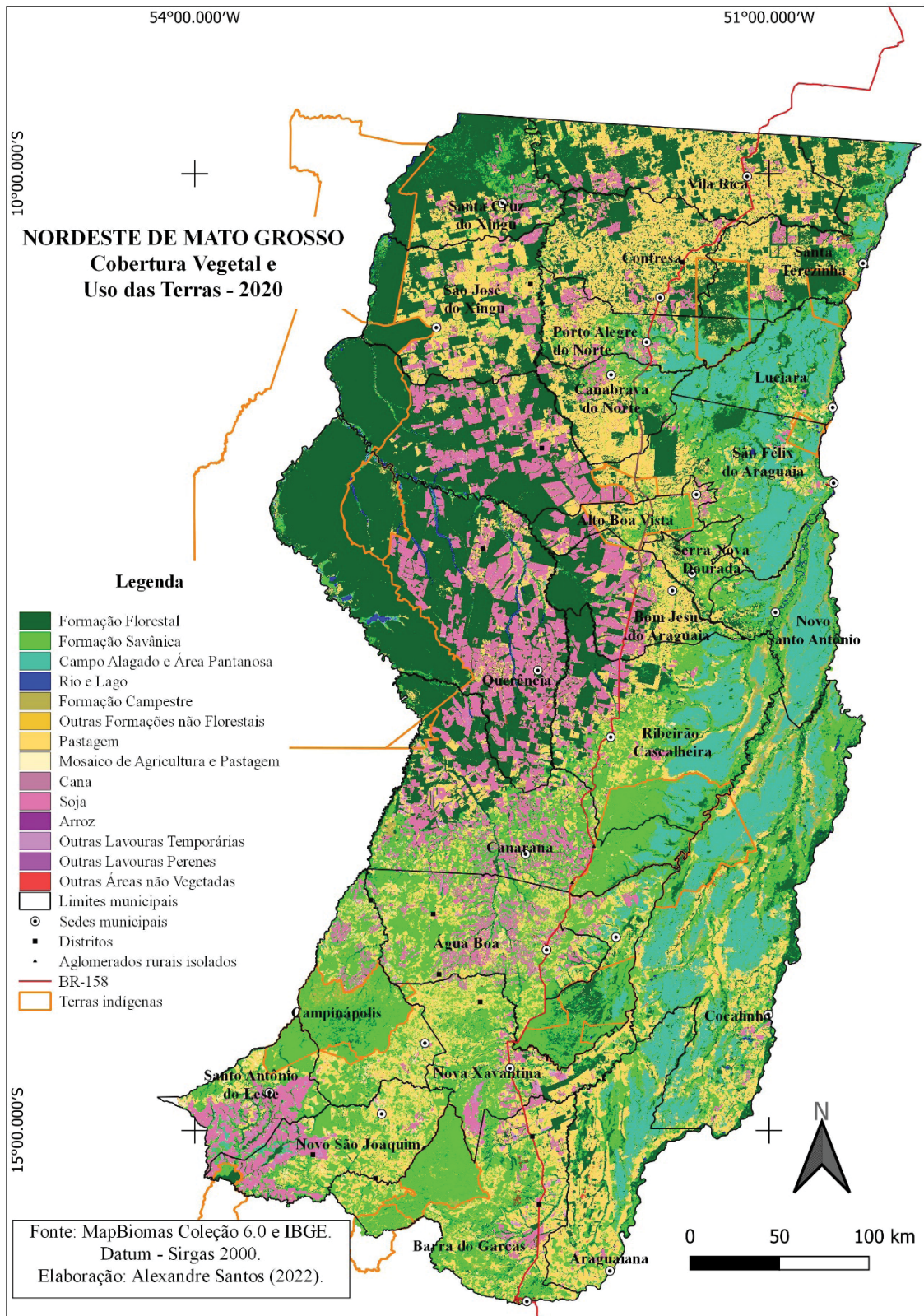
Figura 6 – Mapa da Cobertura Vegetal e Usos das Terras no Nordeste de Mato Grosso em 2020.
