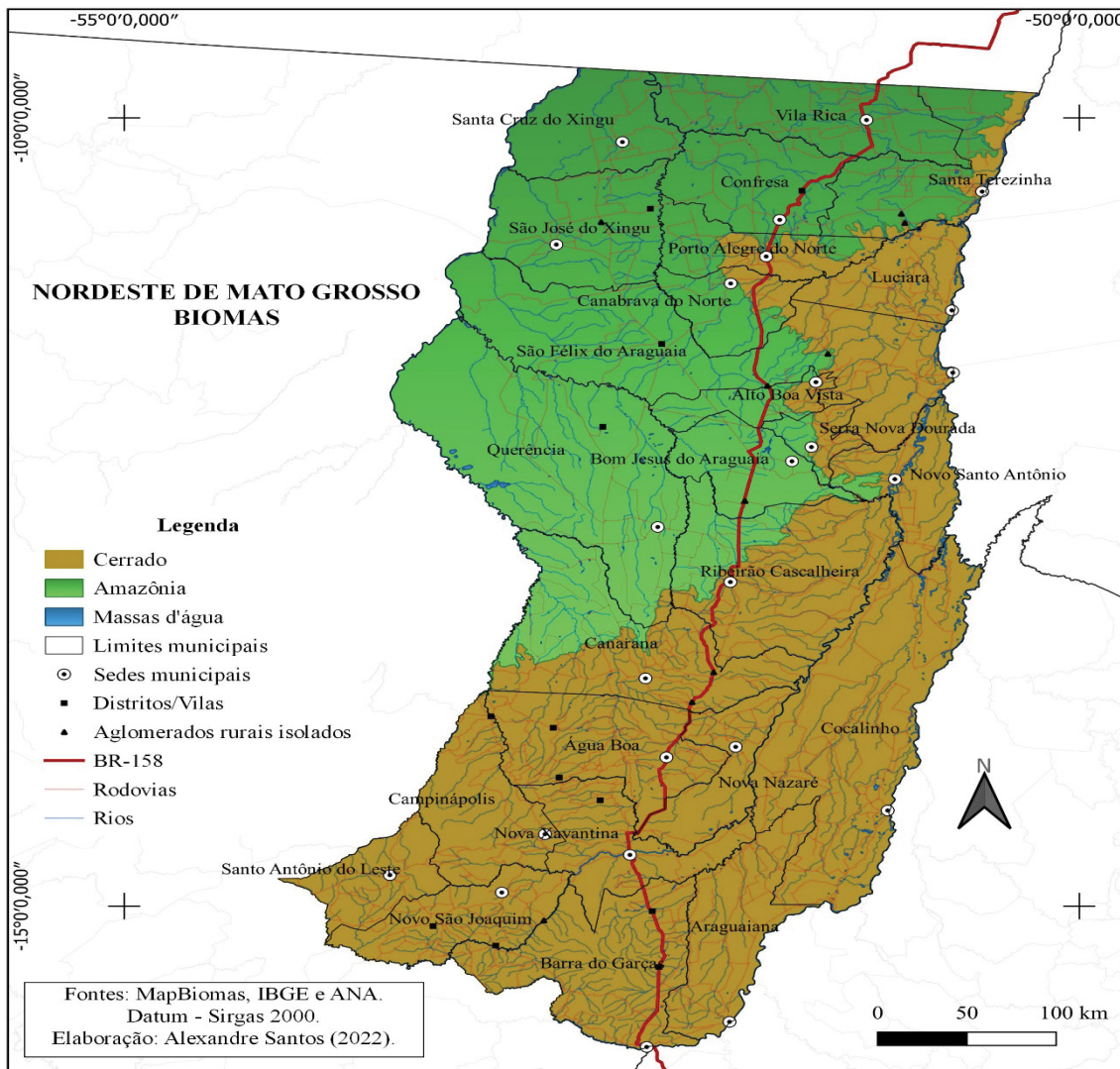
Figura 2 – Mapa dos Biomas do Nordeste de Mato Grosso.
