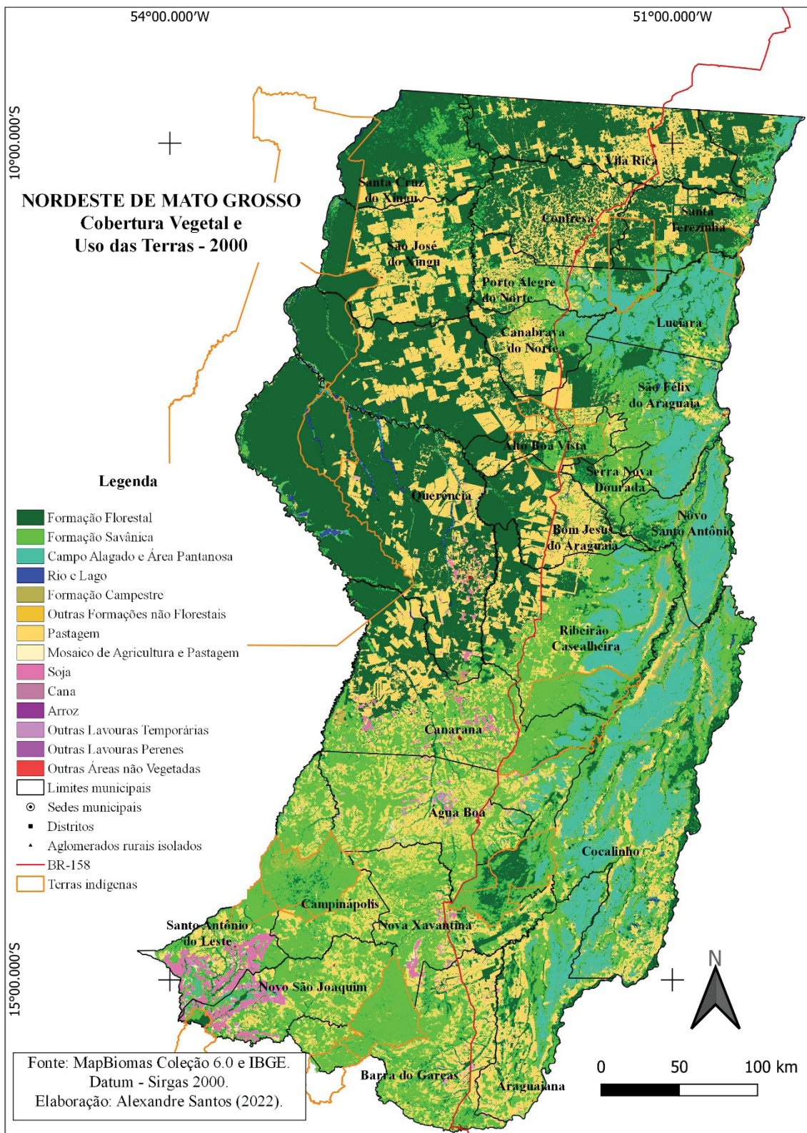
Figura 5 – Mapa da Cobertura Vegetal e Usos das Terras no Nordeste de Mato Grosso em 2000.
