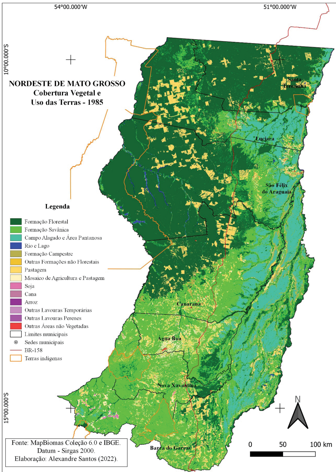
Figura 4 – Mapa da Cobertura Vegetal e Usos das Terras no Nordeste de Mato Grosso em 1985.
