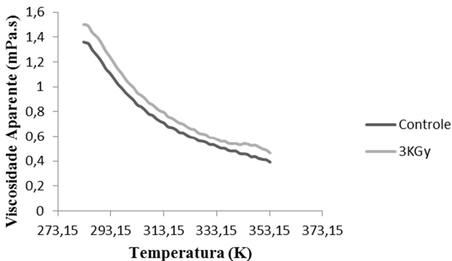
Figura 4. Viscosidade Aparente X Temperatura(K).
