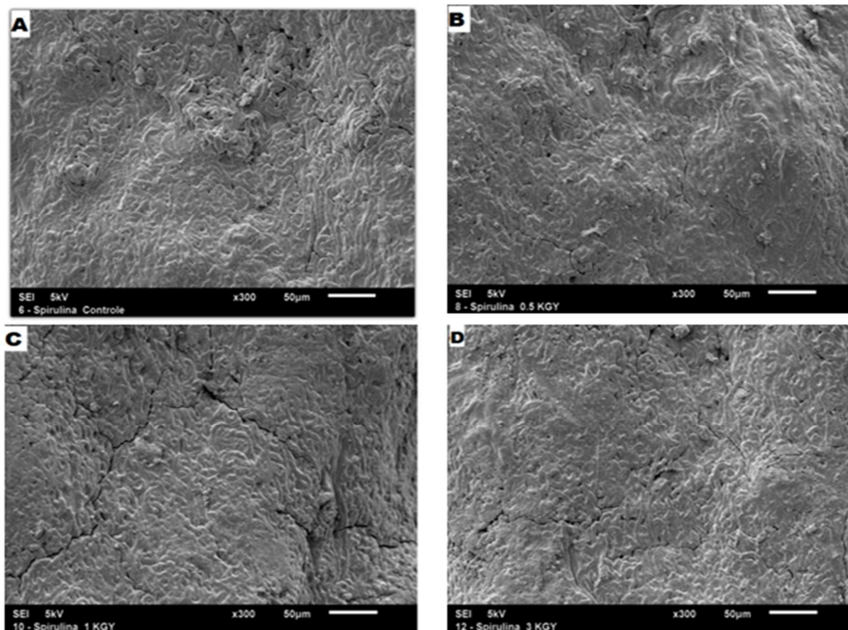
Figura 1. Microscopia eletrônica de varredura da Spirulina submetida à dose de 0(a); 0,5(b); 1,0(c) e 3,0(d)kGy.
