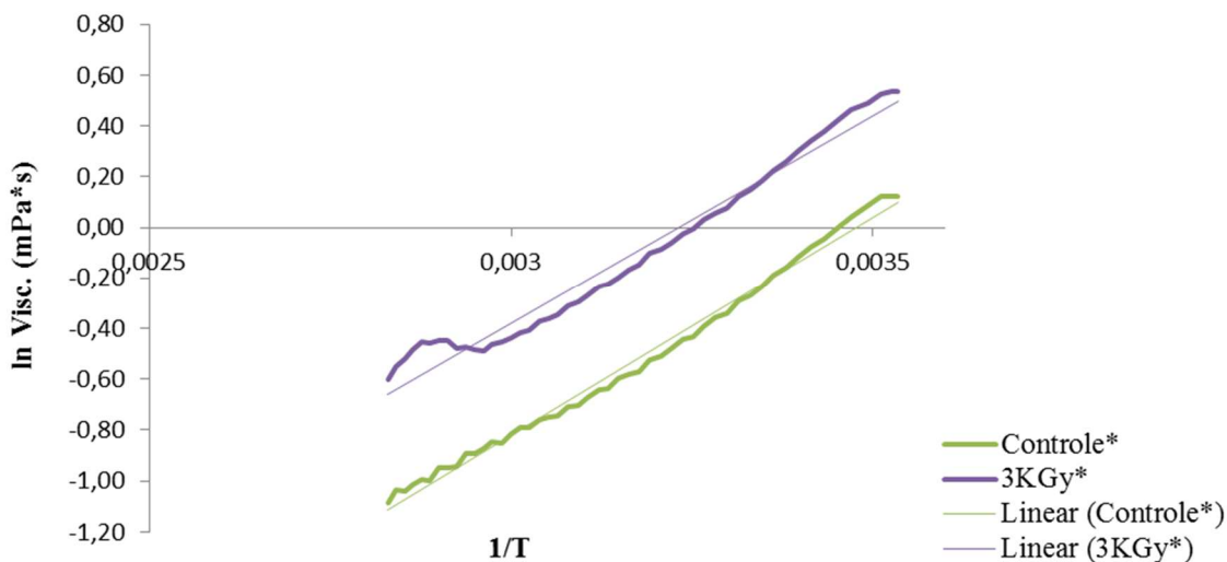
Figura 5. Gráfico de \ln \mu \times 1/T – de acordo com a equação de Arrhenius.
